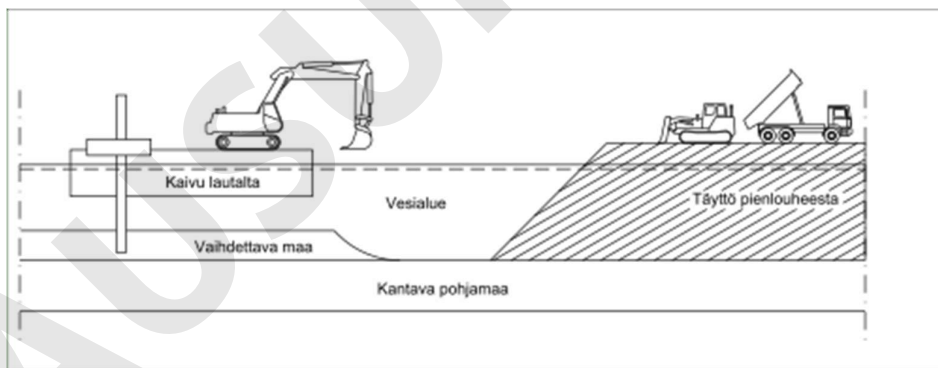
Kuva 16250.K3. Vedenalainen massanvaihto.
