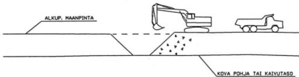
Kuva 16250.K2. Massanvaihto kaivantoon penkereen päältä kaivuna
