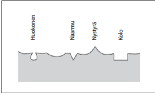
Kuva 1 Havainnekuva alustasta ennen esi- ja pintakäsittelyjä.
